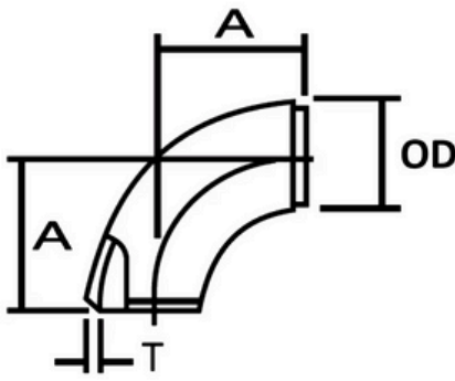
90° Elbow long radius
