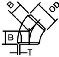
45° Elbow
